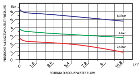
CURVE DI PORTATA*FLOW CHARTS
