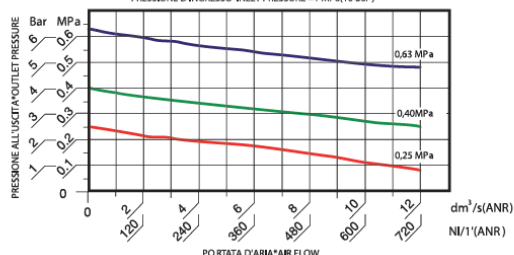
CURVE DI PORTATA*FLOW CHARTS
